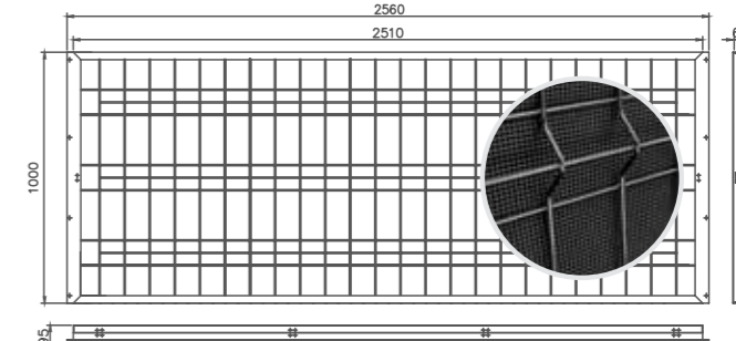
Vorderseite 3D Gitter
